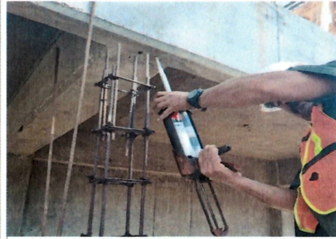
1.- ANCLAJE QUÍMICO
